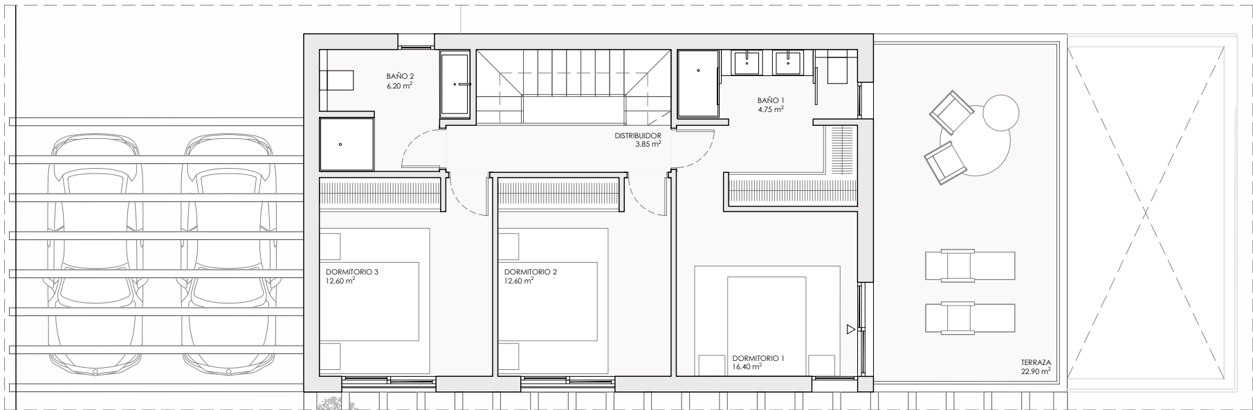
PLANTA PRIMERA
