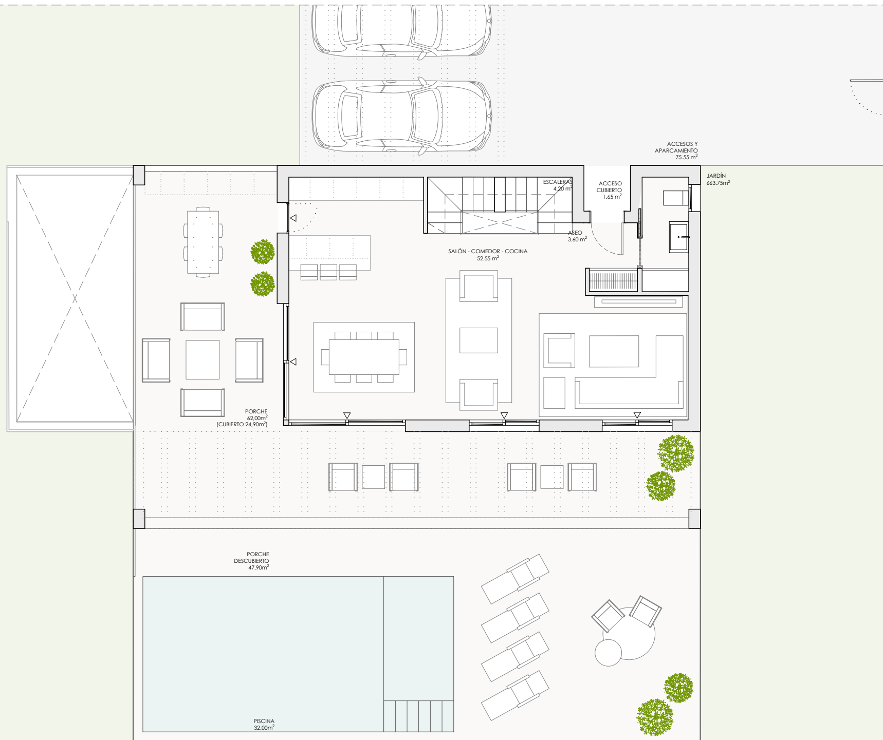
PLANTA BAJA (TIPO A)
